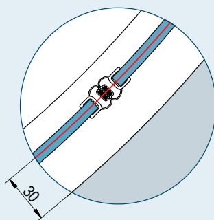
Obr. 3: Při montáži na vaničku je odsazení 30 mm stejné pro standardní i zvláštní rozměry.
