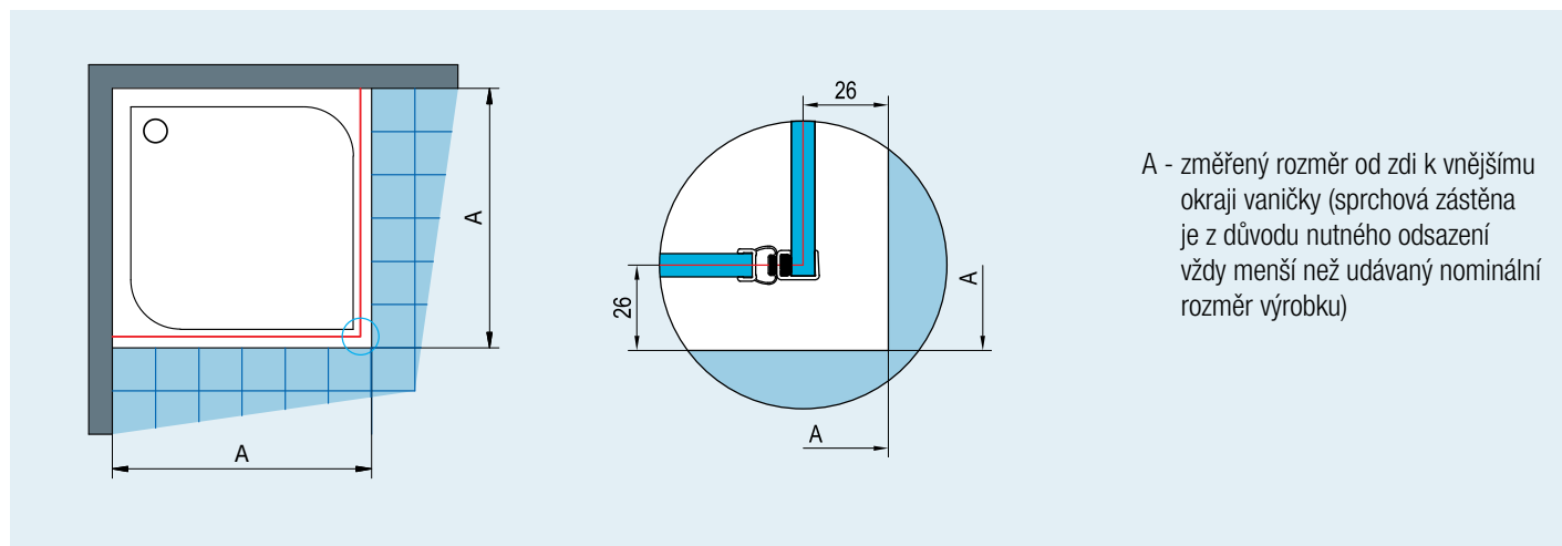
Obr. 1 Při montáži na vaničku je odsazení 26 mm stejné pro standardní i zvláštní rozměry.
