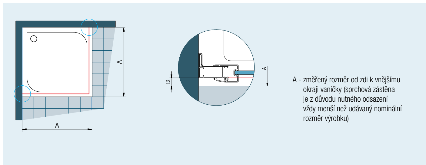
Obr. 1: Při montáži na vaničku je odsazení 13 mm stejné pro standardní i zvláštní rozměry.
