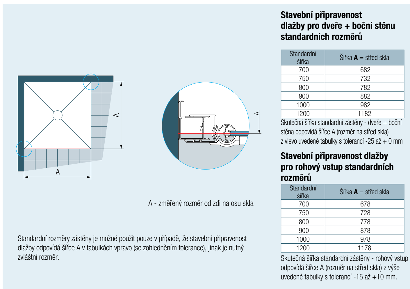
Obr. 2: U montáže na dlažbu se při výrobě nezohledňuje žádné odsazení
