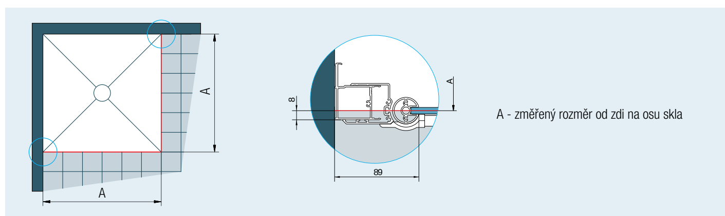
Obr. 2: U montáže na dlažbu se při výrobě nezohledňuje žádné odsazení
