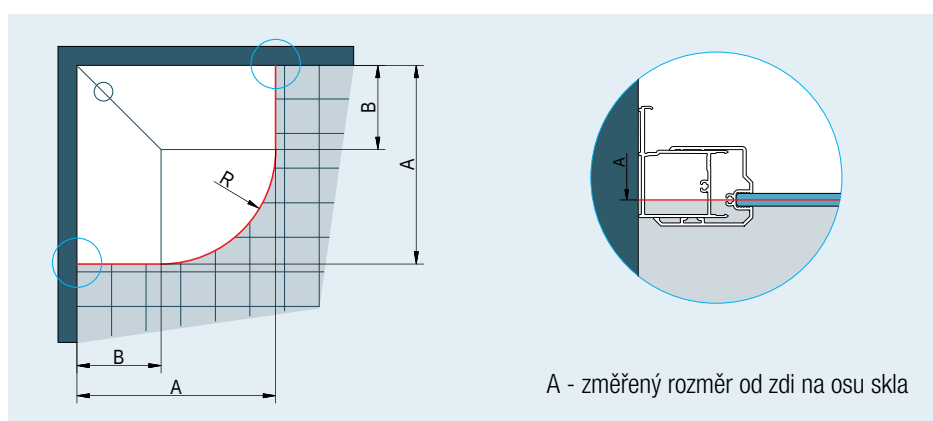
Obr. 4: U montáže na dlažbu se při výrobě nezohledňuje žádné odsazení. U dlažby je nutné zohlednit rádius R477 nebo R527 (viz tabulky vpravo).
