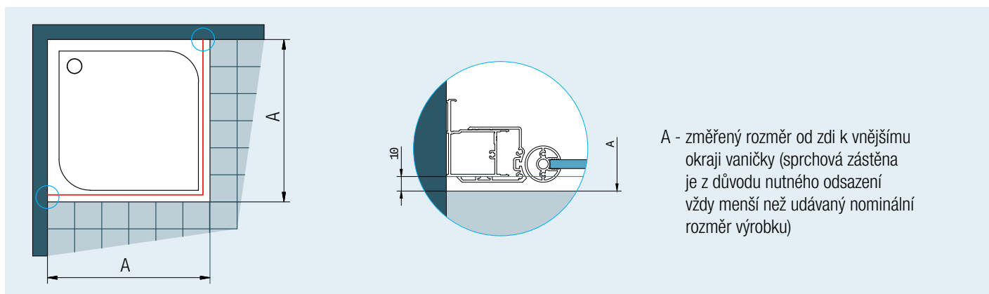
Obr. 1: Při montáži na vaničku je odsazení 10 mm stejné pro standardní i zvláštní rozměry.
