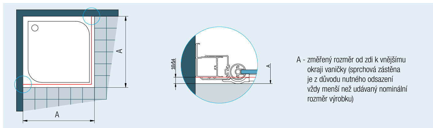
Obr. 1: Při montáži na vaničku je u dveří s boční stěnou odsazení 10 mm stejné pro standardní i zvláštní rozměry. U rohového vstupu je odsazení 14 mm.
