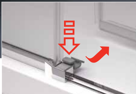
Posuvné díly dveří lze pro snadné čištění jednoduše odklopit.
