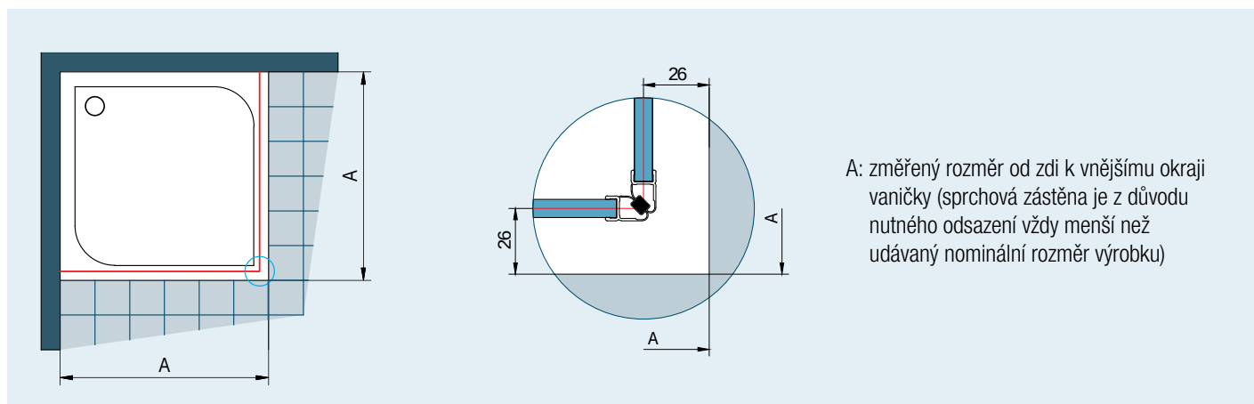
Obr. 1: Při montáži na vaničku je odsazení 26 mm stejné pro standardní i zvláštní rozměry.
