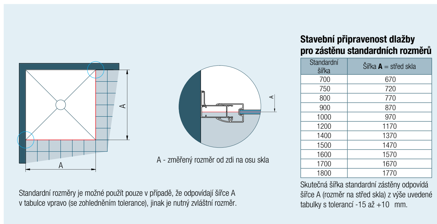
Obr. 2: U montáže na dlažbu se při výrobě nezohledňuje žádné odsazení.
