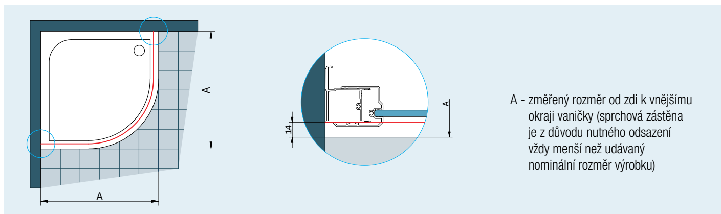
Obr. 3: Při montáži na vaničku je odsazení 14 mm stejné pro standardní i zvláštní rozměry.
