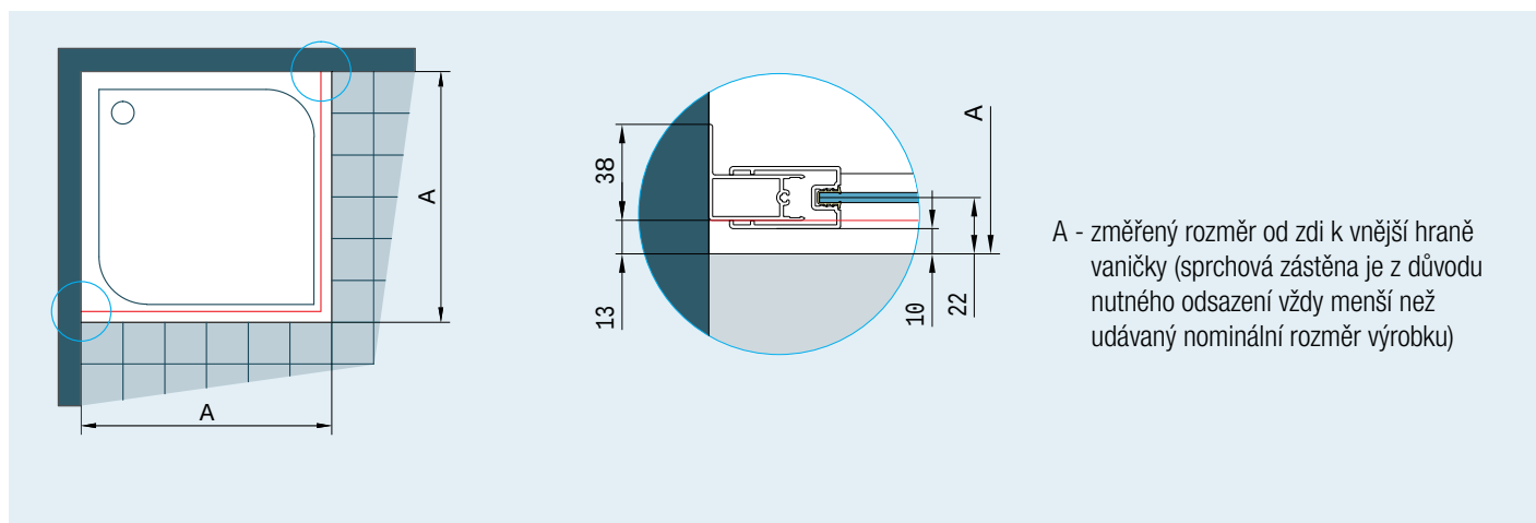
Obr. 1: Při montáži na vaničku je odsazení 13 mm.
