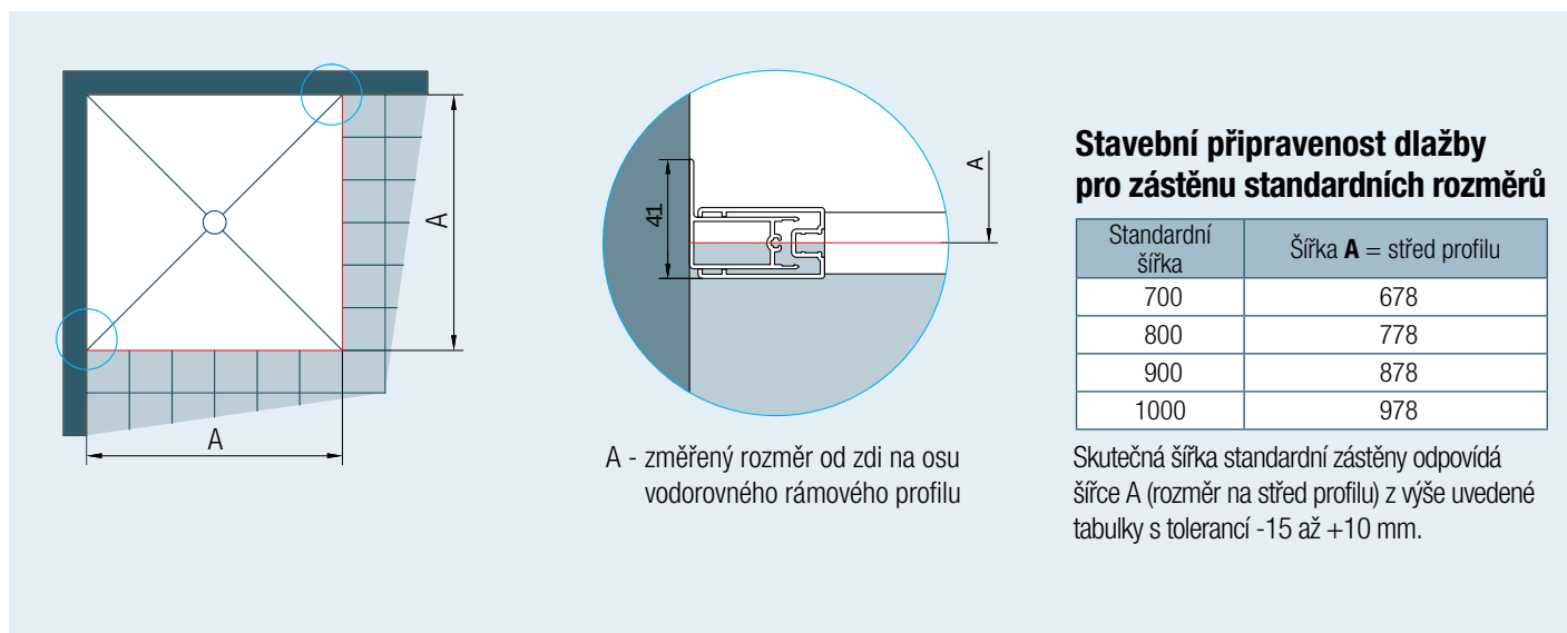
Obr. 2: U montáže na dlažbu se při výrobě nezohledňuje žádné odsazení.
