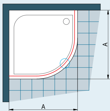
Obr. 3: Při montáži na vaničku je odsazení 30 mm stejné pro standardní i zvláštní rozměry.
