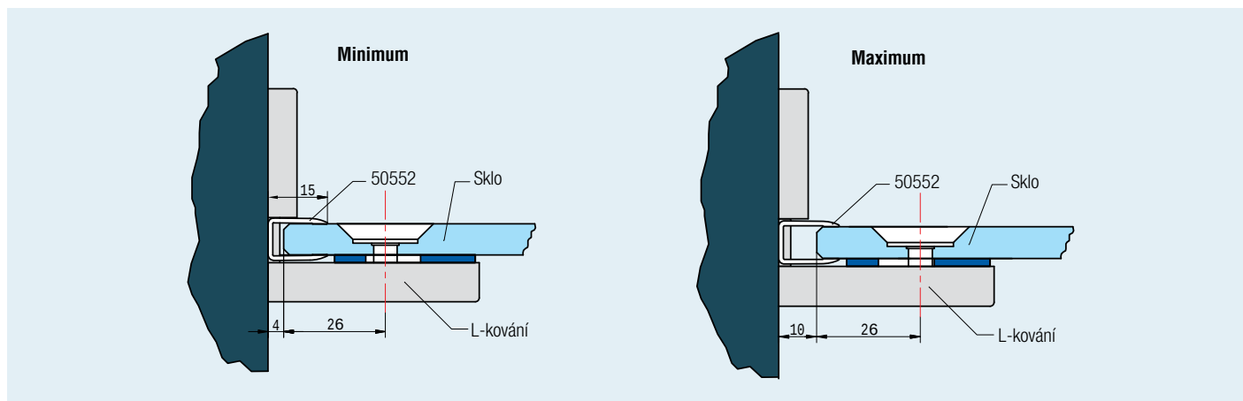
Obr. 5: L-kování s těsnicím U-profilem 50552 umožňuje vyrovnání nerovností zdi do 6 mm. Těsnicí U-profil 50552 umožňuje zakrýt mezeru mezi zdi a sklem.
