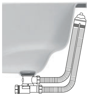
Skrytý vanový odtokový komplet k vaně bez přepadu
