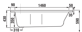
Instalační rozměry vany s panelem
