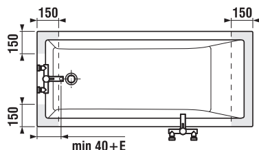
Instalační rozměry vany bez panelu
