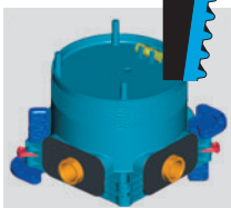
Seřízněte přechnývací část tělesa EASY-Boxu
