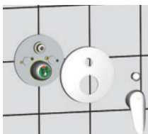
Nasadte rozetu, páku a táhlo přepínače
